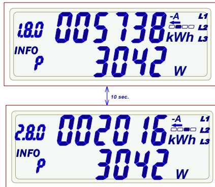
Abb. 8: Anzeige 2- Richtungszähler
